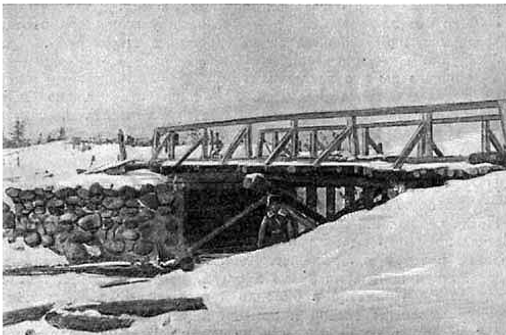
Мост, построенный саперами на месте разрушенного белофиннами
